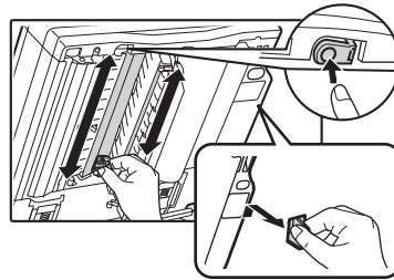
Pappersmatningsrulle
